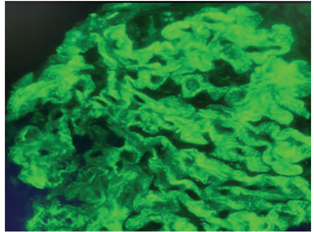
Kappa Stain
